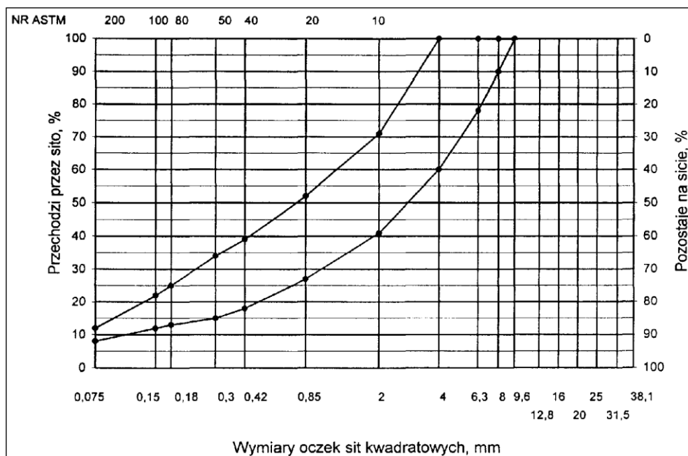
Rys. 3. Krzywe graniczne uziarnienia mieszanki mineralnej BA od 0 do 8mm, od 0 do 6,3 mm do warstwy ścieralnej nawierzchni drogi o obciążeniu ruchem nawierzchni o obciążeniu ruchem KR1 lub KR2
